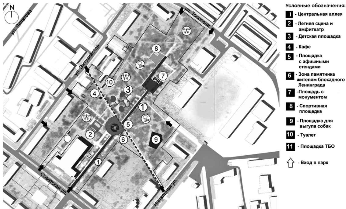
Рис. 2. Схема функционального зонирования (иллюстрация авторов)
