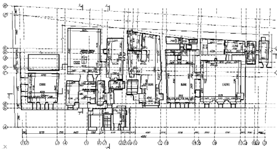
Рис. 4. Схематичный план первого этажа [3, 4]
