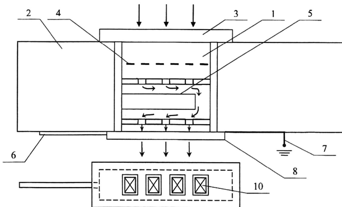
Рис. 1. Устройство приточной вентиляции: вид сверху
