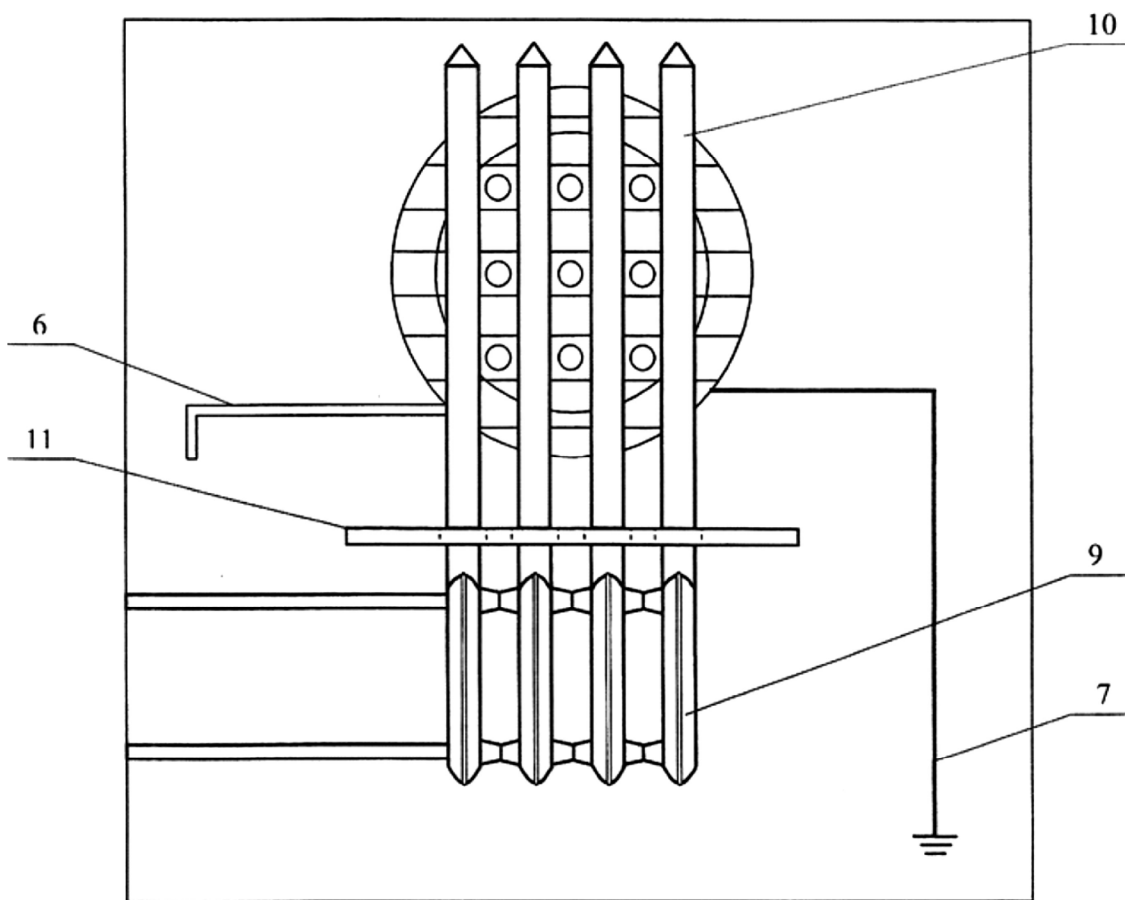
Рис. 2. Устройство приточной вентиляции: вид со стороны помещения
