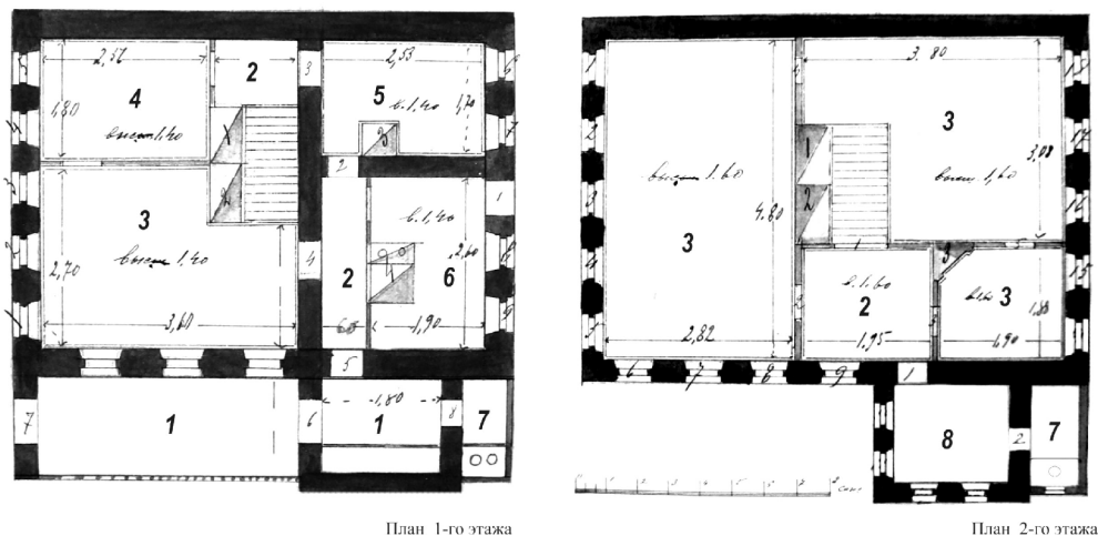
Рис. 2. Планы Петровского (четырнадцатого) городского женского училища в доме Музурова на ул. Георгиевской. Кон. XIX – нач. XX вв. 1. Вход. 2. Коридор. 3. Классы. 4. Класс для рукоделия. 5. Библиотека. 6. Комната сторожа. 7. Туалет. 8. Рекреация.
