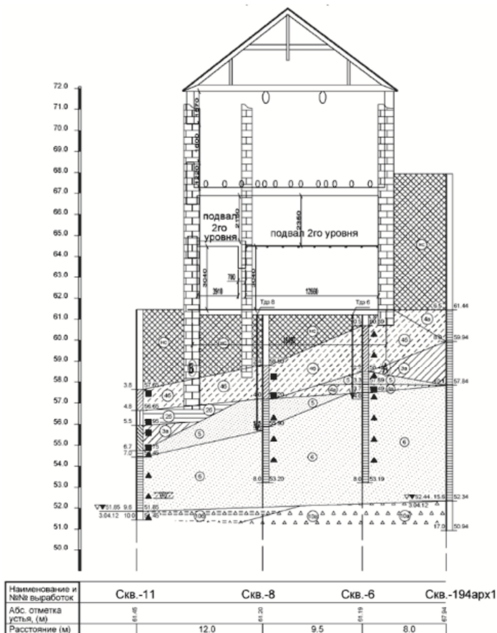
Рис. 3. Совмещенный геологический разрез и разрез по зданию [1]
