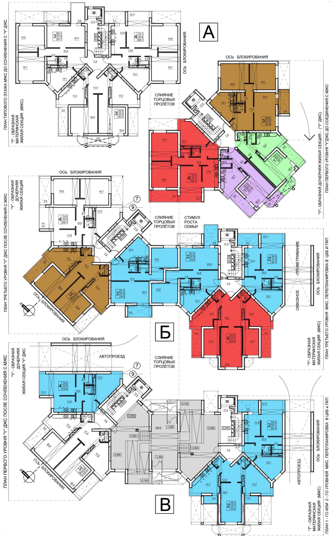
Рис. 4. Схема парного соединения секций №№ 01 и 02; 08 и 09. (Иллюстрация автора). Fig 4. Scheme of pair connection of sections No. 01&02; 08 &09. (Illustration by the author)
