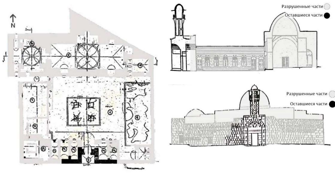
Рис. 5. Фрагменты уцелевшей части медресе на плане, фасаде и разрезе школы Аль-Султанья после войны (чертежи авторов)
