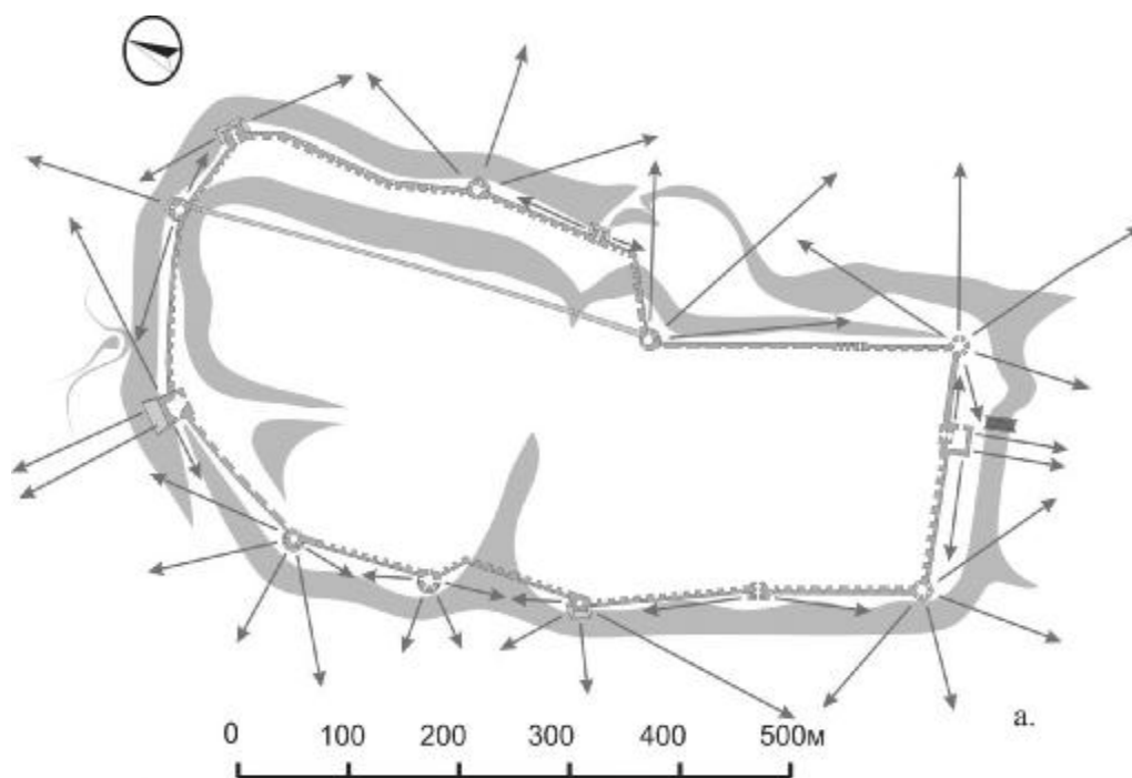
Рис. 3. Схема комбинации различной формы башен в Казанском кремле (схема с указанием зон обстрела фланкирующим огнем на уровне бойниц подошвенного боя)
